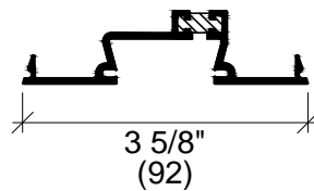
F2004 MULLION / SILL FILLER
